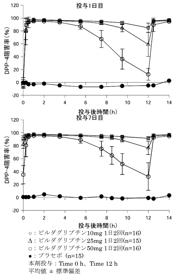
2 型糖尿病患者にビルダグリプチン 10、25、50mg を 1 日 2 回、7 日間反復投与したときの投与 1 日目と 7 日目の DPP-4 阻害率の推移
